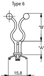
Diam. trou: Voir detail Fig. 6 Épaisseur: 0.8-1.6
